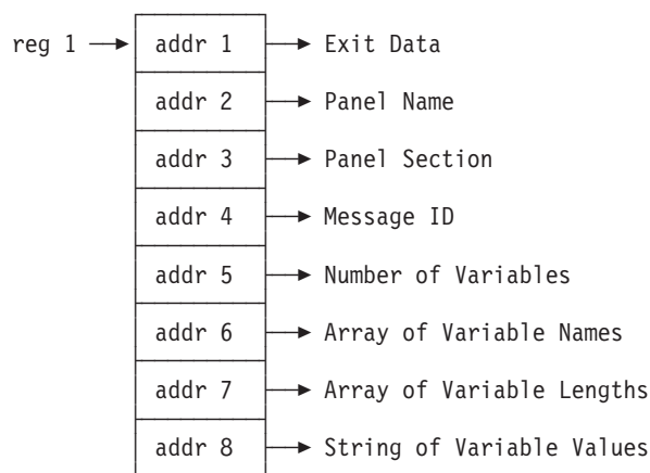
Figure 69. Standard parameter list format
